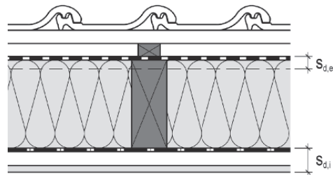
Bild 16. Definition der inneren ( s_{d,i} ) und äußeren ( s_{d,e} ) wasserdampfäquivalenten Luftschichtdicke ( s_d -Wert); gestrichelte Linie: unter der Unterdeckbahn kann sich bspw. noch eine Holzschalung befinden
