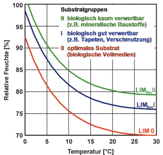
Bild 4. Grenzkurven für das Auskeimen von Schimmelpilzsporen (Isolethen) für unterschiedliche Substrate. Unterhalb dieser Grenzkurven (LIM = Lowest Isoleth for Mould), die eine einhüllende Funktion für alle baurelevanten Schimmelpilzspezies darstellt, findet keine Sporenauskeimung und damit auch kein Schimmelpilzwachstum statt.
