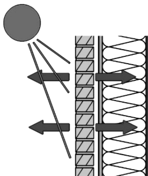
Bild 3. Bei Besonnung einer regenfeuchten Mauerwerks-vorsatzschale entsteht durch die Erwärmung des Mauerwerks ein Dampfdruckgefälle in beiden Richtungen, das dazu führt, dass während der Austrocknung ein starker Dampfdiffusionsstrom auch in die Holzkonstruktion stattfindet. [2]
