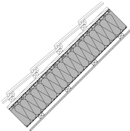
Bild 20. Sanierendes Altbaudach
