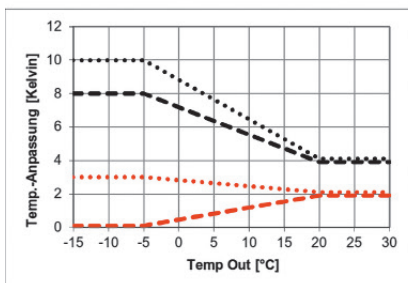
Bild 11. Ableitungskurven für Temperatur und Luftfeuchte in unbeheizten Dachräumen aus dem Außenklima für folgende bauliche Bedingungen:
