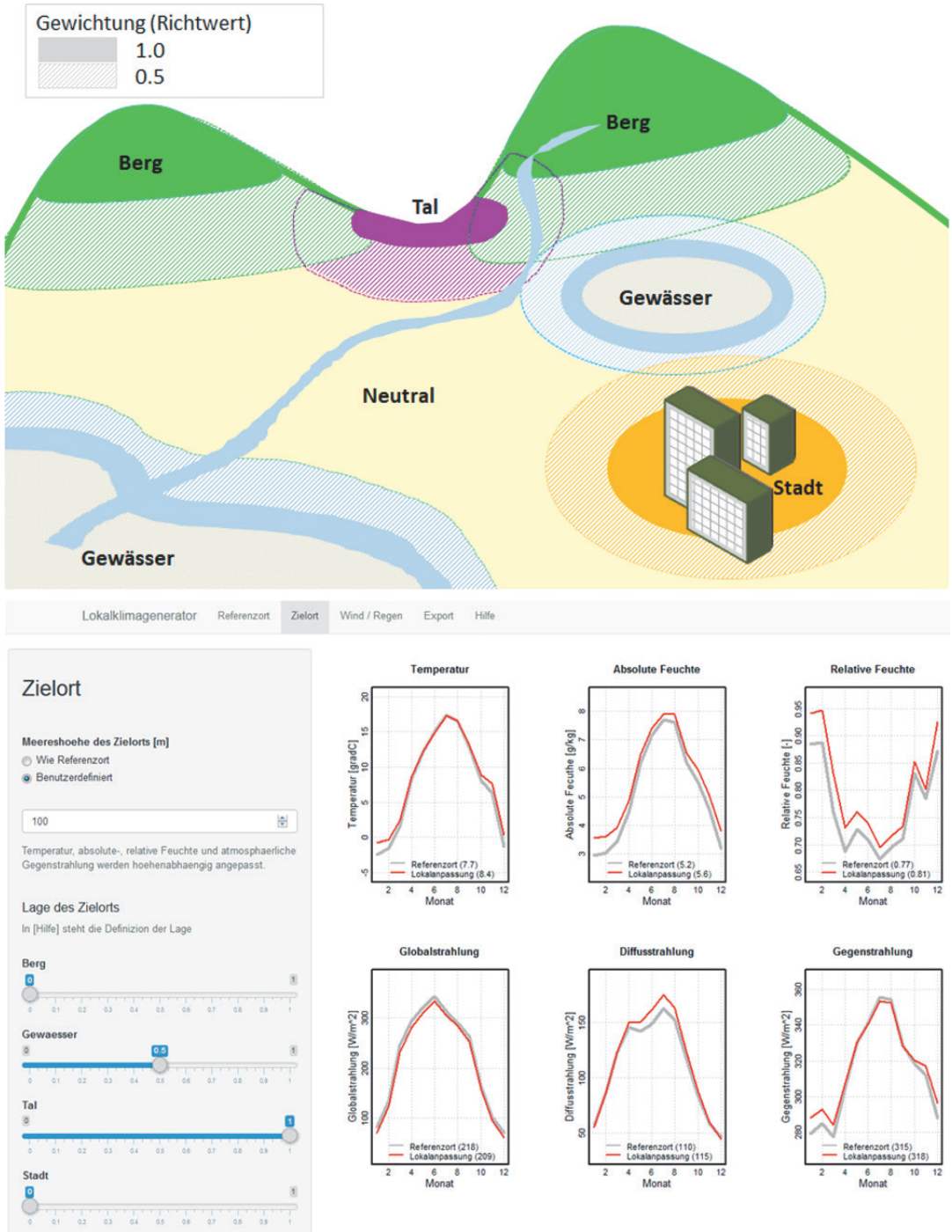
Bild 10. Anpassung Klimaverhältnisse auf die lokalen Bedingungen auf Basis des regionalen Referenzklimadatenatzes mithilfe des Lokalklimagenerators gem. [72, 73]
